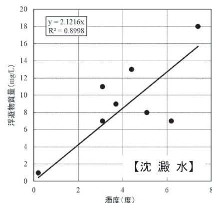
検討結果例(濁度とSSの関係)
