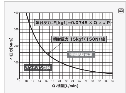
噴射反力グラフ
